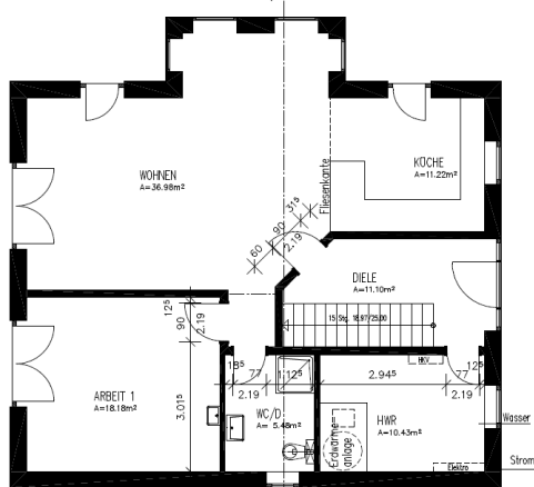
EG Bauherren-Grundriss
