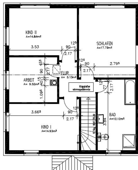
DG Bauherren-Grundriss
