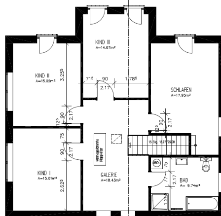
DG Bauherren-Grundriss
