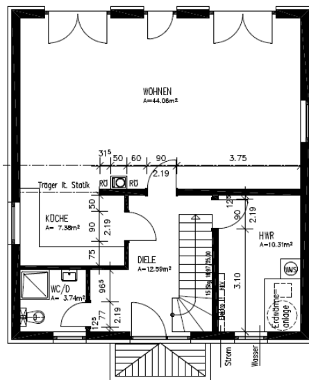
EG Bauherren-Grundriss
