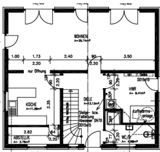
Erdgeschoss MICHENDORF
