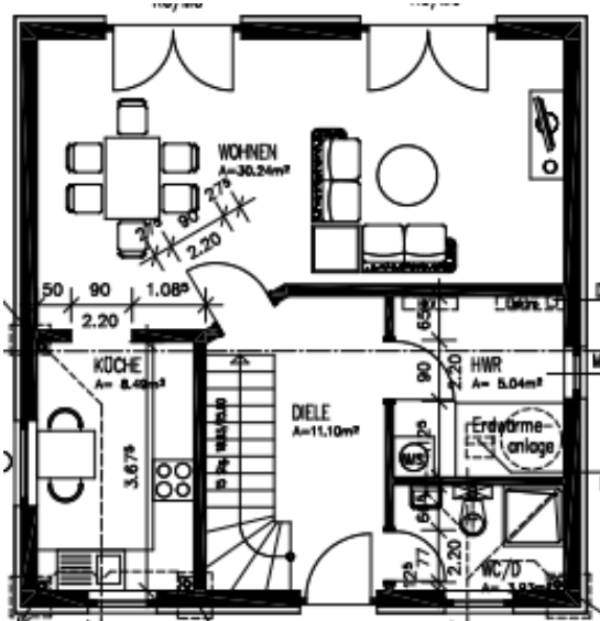
Erdgeschoss MICHENDORF
