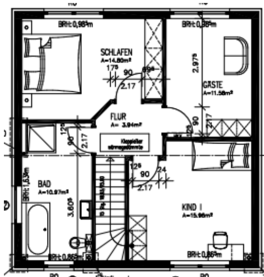
Obergeschoss MICHENDORF
