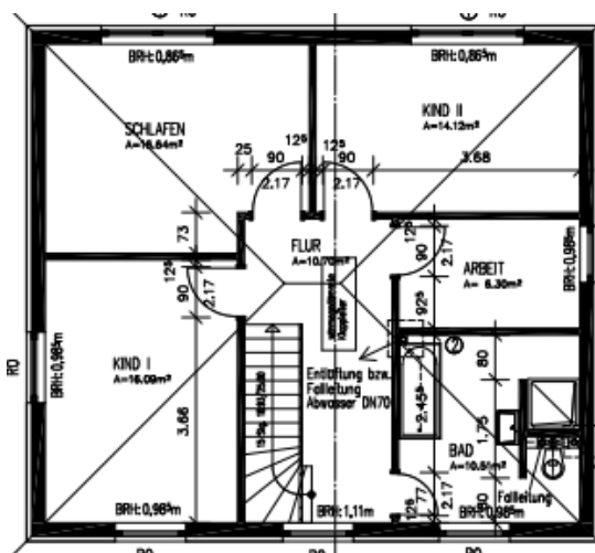
Obergeschoss MICHENDORF
